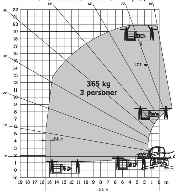
ROTATION PÅ STØTTEBEN FULDT UDSKUDT MED UDSKYDELIG PLATFORM 2,25/4 m
